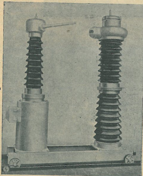
Egysarkú 100.000 voltos szabadtéri expanziós kapcsoló, 10.000 ampère kikapcsolására.
