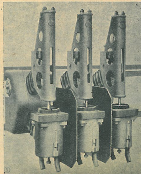
Háromsarkú, 10.000 voltos expanziós kapcsoló, 15.000 ampère kikapcsolására.
