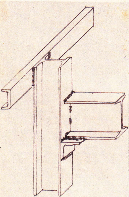
Ívlánggal hegesztett vasszerkezet
