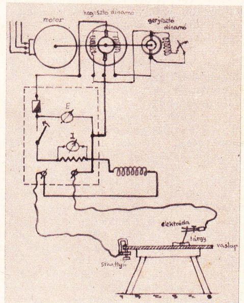
Hegesztődinamó kapcsolási vázlat
