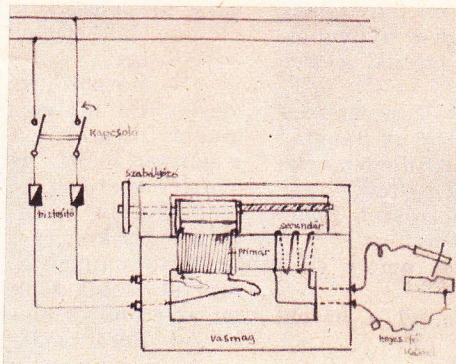
Hegesztőtranszformátor kapcsolása
