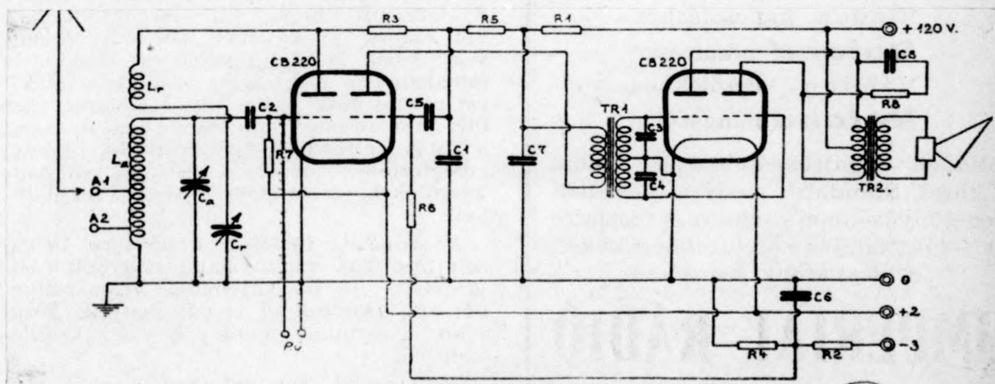
A kétlámpás telepes Európavevő kapcsolási rajza
