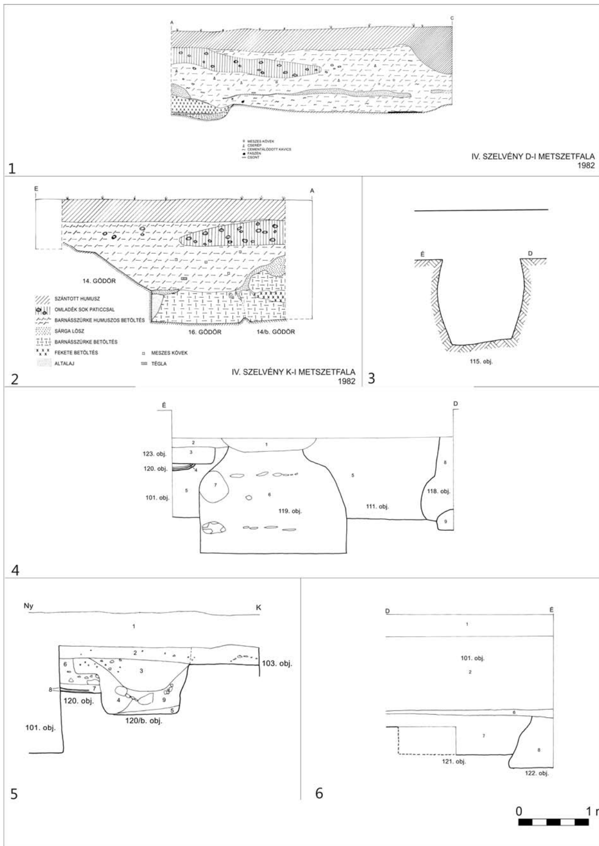
VII. tábla: Objektumrajzok, metszetrajzok
