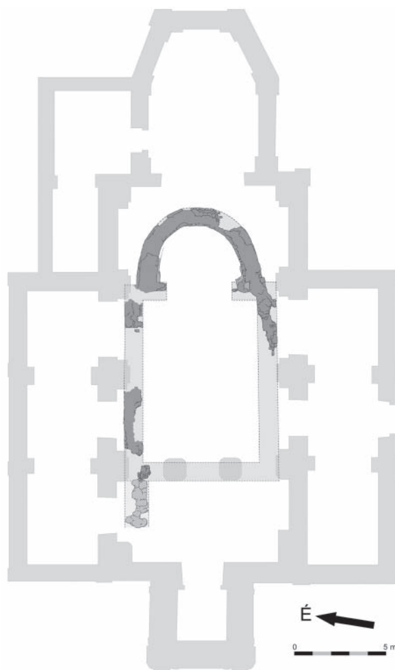
4. ábra. Karád, a középkori templom kiszerkesztett alaprajza, a mai környezetbe vetítve.
