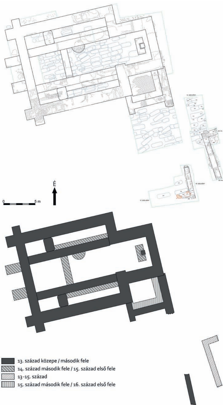
1. ábra. Bárdudvarnok, a feltárások összesített alaprajza (2014-2017, 2019) és a monostori templom építési fázisai.
