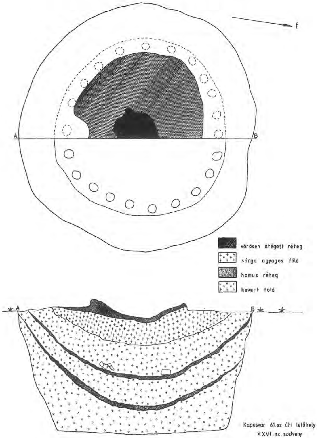
38. ábra: Cölöpös építmény metszetrajzai (Rajz: Bajóné Sótónyi Mária)
