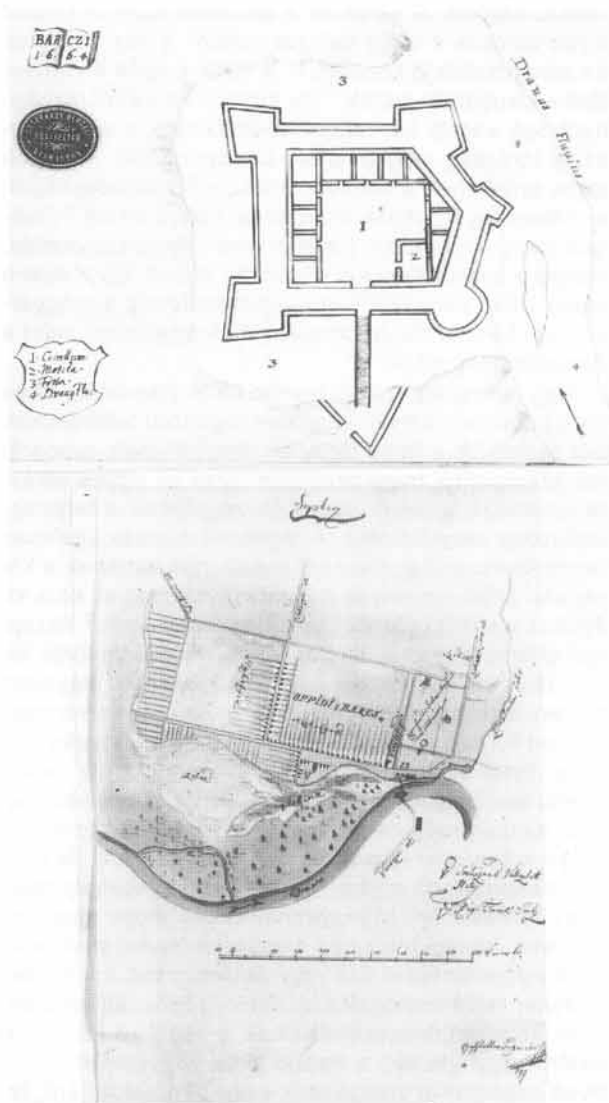
2. a) Az 1664. évi Esterházy-féle váralaprajz. b) Az 1799. évi felmérés a vár helyének megjelölésével
