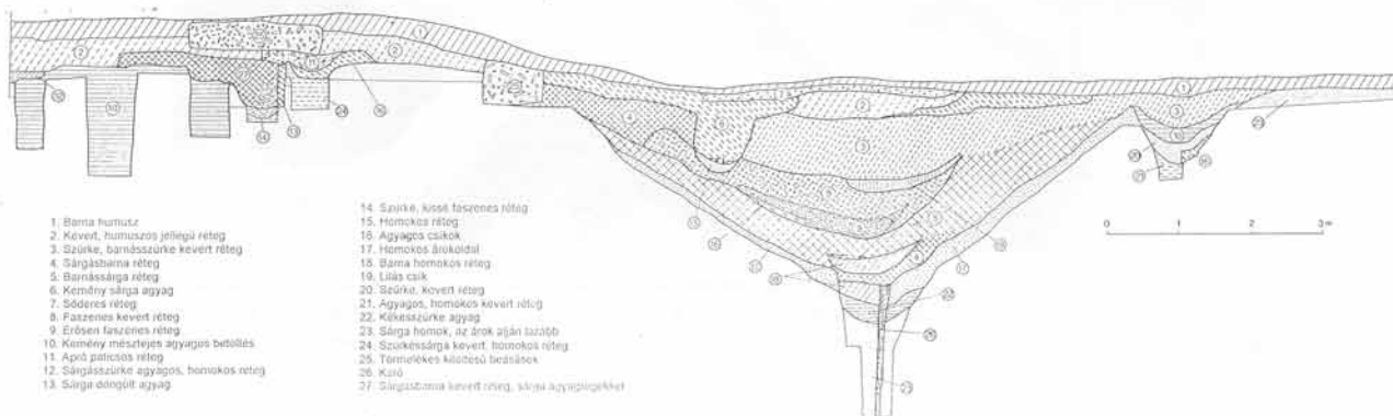
10. A vár erősítési rendszerének egy metszete a várárokkal és a palánkmegújításokkal (ÁI/94)
