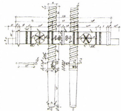
Ikerorsós szőlőprés Kisillés Sándor pincéjéből Sási János felmérési rajza, 1983
