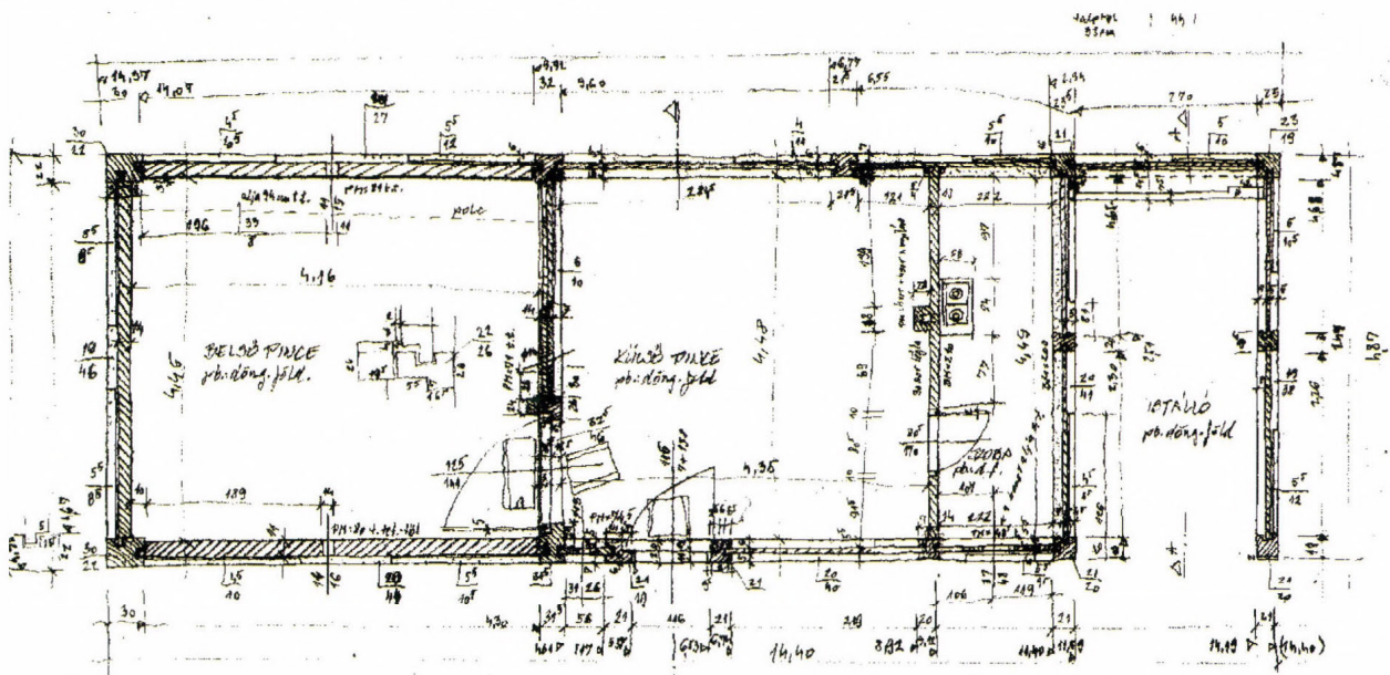
Kisillés Sándor pincéje az alsősegesdi szőlőhegyről Sási János felmérési rajza, 1983
