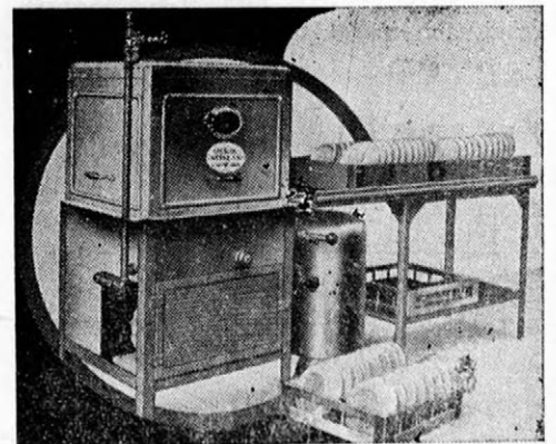
Önműködő edénmosogató
