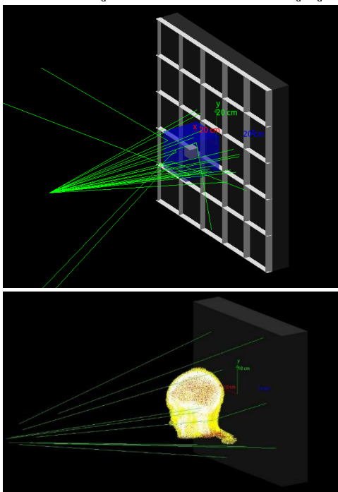
6. ábra: Röntgengépek sugárzásának csökkentése Geant4 szimulációkkal. Forrás: a Szerző
