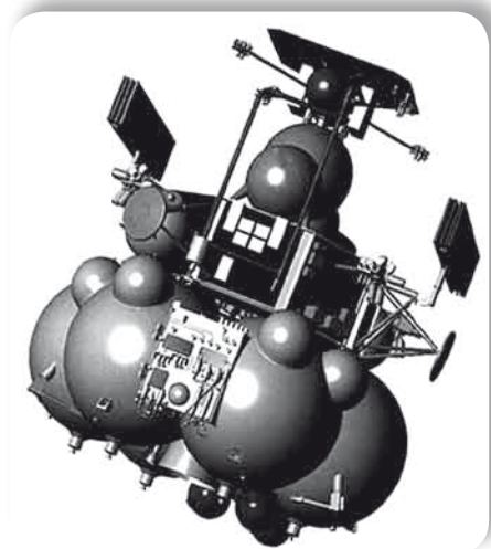
A Fobosz-Grunt szonda
