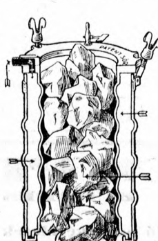
A készülék hosszszetszete.
