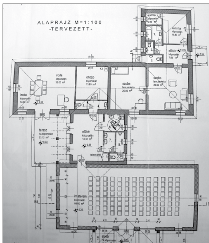
A tervrajz felső része a már meglévő és átalakítandó, az alsó az új épületrészt tartalmazza
