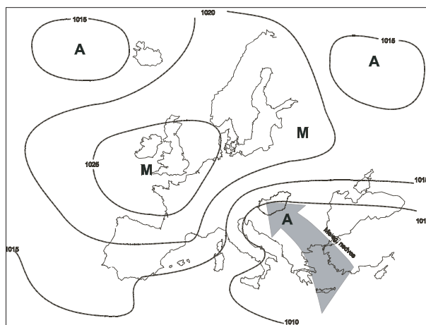
9. ábra: 2005. nagy csapadékos helyzeteinek jellegzetes nyomási képe a meleg, nedves szállítószalaggal
