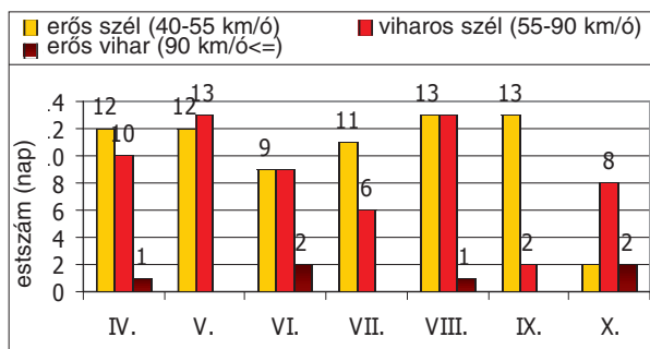
2. ábra A napi maximális széllelőkések alakulása a 2006. évi viharjelzési szezonban a Balatonnál
