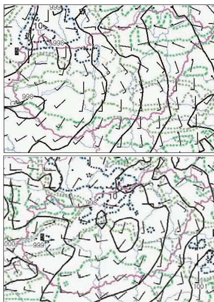
5. ábra Az ALADIN.HU modell által előrejelzett légnyomás és szél adatok 2006. 02. 17-én 09 és 12 UTC-kor, valamint csapadékmennyiség adatok 06 és 09, valamint 09 és 12 UTC között Folytonos vonal: nyomás – Szélzászlók – Szaggatott vonal: csapadék (vastag: 5 mm felett)
