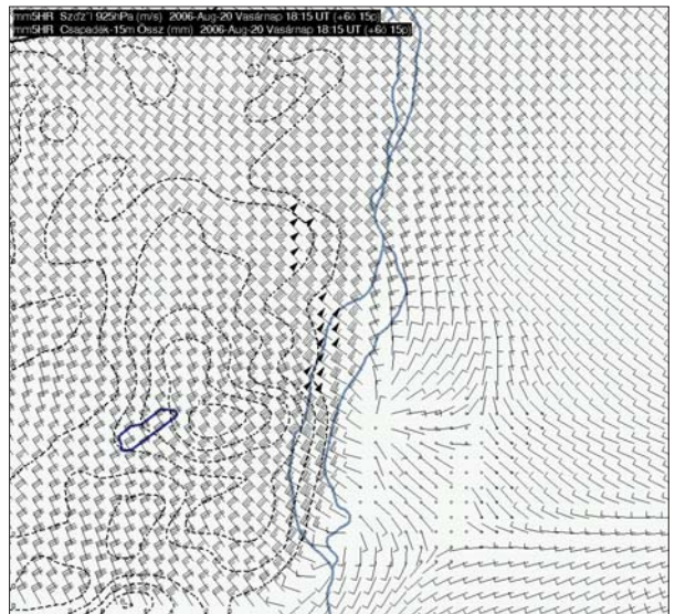
8. ábra. Az MM5 modell 18:15 UTC-re vonatkozó 925 hPa-os előrejelzett szélmezeje és a 15 perc alatt lehullott csapadék mennyisége (szaggatott vonal).
