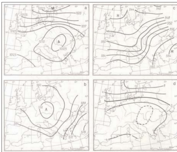
2. ábra: Centrum típusú időjárási helyzet a/ közepes talajmenti nyomásmezeje, b/ közepes 500 hPa-os felülete, c/ közepes 500/1000 hPa-os rétege, d/ közepes eltérése a normál értéktől a talajon
