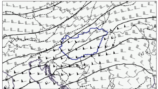
2. ábra. Az 500 hPa-os szint magassága (folytonos vonal), hőmérséklete (szaggatott vonal) és szele 2006. augusztus 20. 18 UTC-kor az ECMWF +6 óras előrejelzése alapján.
