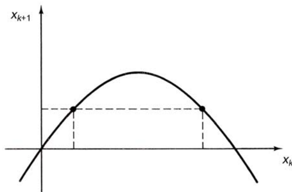
1. ábra. A logisztikus leképezés neminvertálható jellege.
