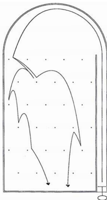
3. ábra. A tivoli csaknem egyforma sebességgel kilőtt két golyója által követett pálya.
