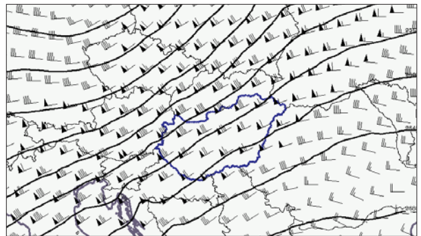
3. ábra. A 300 hPa-os szint magassága (folytonos vonal) és szélmezeje 2006. augusztus 20. 18 UTC-kor az ECMWF +6 óras előrejelzése alapján.
