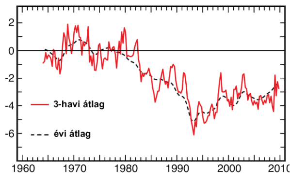
1. ábra: A globális teljes ózonnemennyiség változása az 1964-1980 közötti átlaghoz képest (%) (Fahey and Hegglin, 2011)
