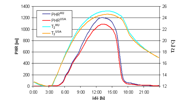
3. ábra: A PHR magasság és a T_2 modellterületi átlagának időbeli változása magyar (HU) és az egyesült-államokbeli (USA) talajok esetén 2009. 07. 13.-án.
