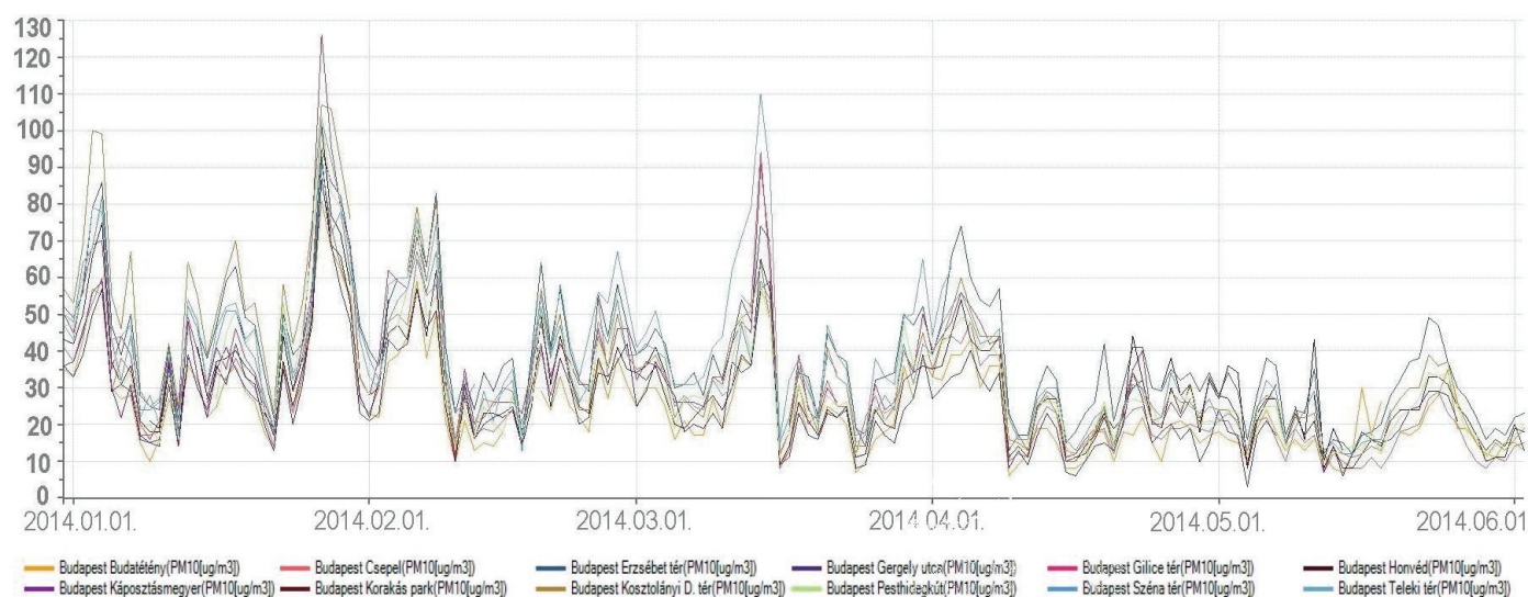
5. ábra: Budapest mérőállomásain mért PM_{10} szennyezettség
