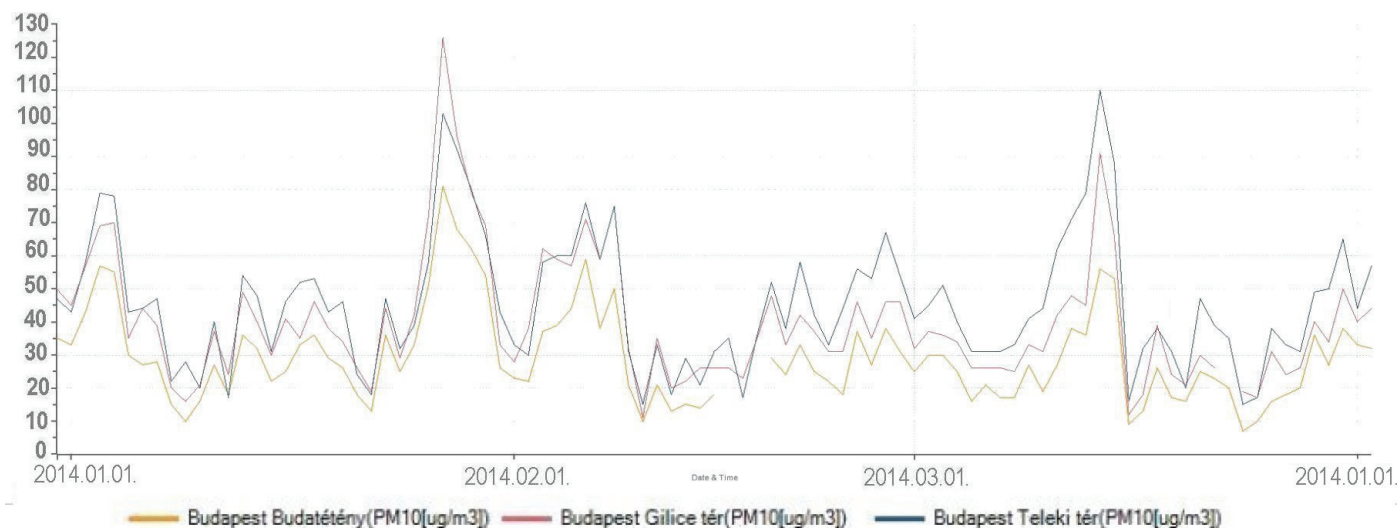
6. ábra: Két városi háttér (Budapest, Gilice tér és Budapest Budatétény) és egy közlekedési állomás (Budapest, Teleki tér) PM_{10} mérési adatai (órás átlag)
