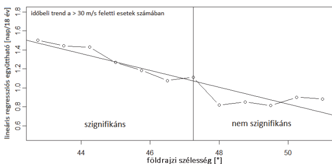
5. ábra: A 250 hPa nyomási szinten előforduló 30 \text{ ms}^{-1} feletti szélsőségek gyakoriságának csökkenését jelző lineáris regressziós együtthatók (meredekség) abszolút értéke (negatív értékek) a k. h. 18,75^\circ hosszúsági kör mentén
