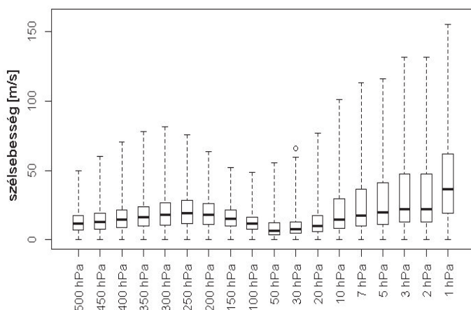
1. ábra: A vizsgált nyomási szintek szélebségeinek gyakorisági eloszlásait reprezentáló Box-Whisker diagram az 1979–2015 időszakra a Budapesthez legközelebb eső rácspont esetében (é. sz. 47,25°, k. h. 18,75°)
