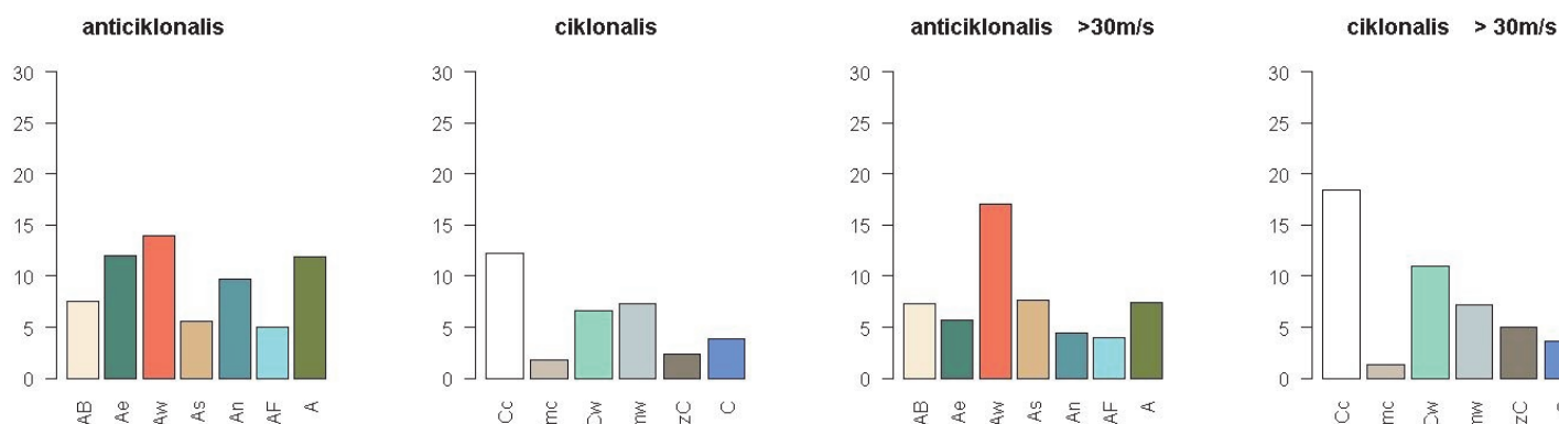
6. ábra: A Péczy-féle makroszinoptikus típusok relatív gyakorisága (%) a teljes 1979–2015 időszakra nézve (bal oldal), illetve azokban az esetekben, amikor a 250 hPa szinten 30 \text{ ms}^{-1} feletti szélsőség figyelhető meg (jobb oldal). Az elemzés a Budapesthez legközelebb eső rácspontra (é. sz. 47,25^\circ , k. h. 18,75^\circ ) készült.
