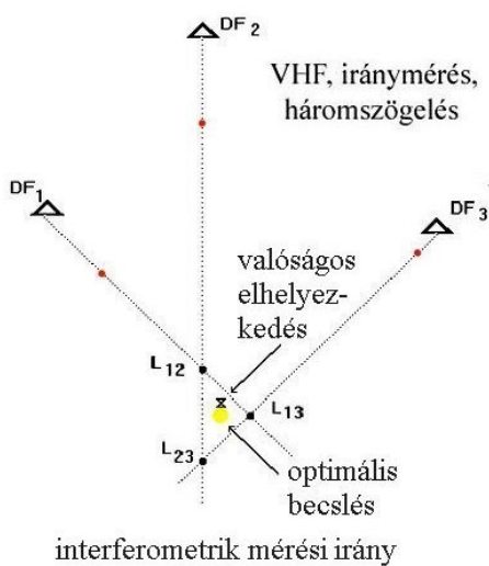
53. ábra: Háromszögeléses mérési módszer
