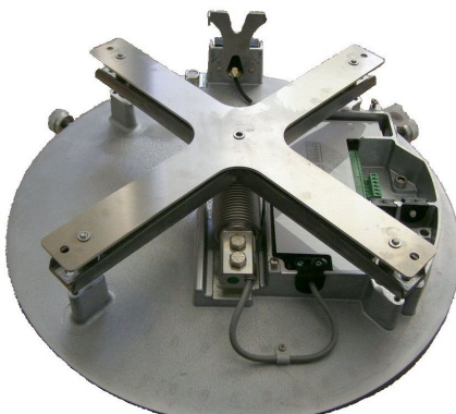
12. ábra: OTT Pluvio csapadékmérő belseje
