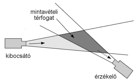
46. ábra: Előreszóródásos mérés elve
