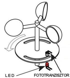
22. ábra: Forgókanalas szélesség mérés elve
