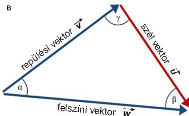
23. ábra: Ultrahangos szélességmérés elve.
