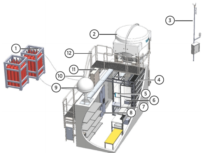
1. ábra: Az AS41 autoszonda rendszer sematikus vázlat
