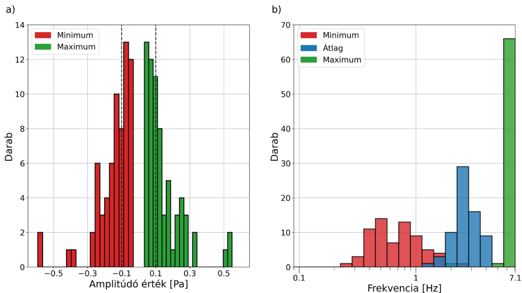
7. ábra. (a) A villámokhoz kapcsolt érzékelések hullámformáiból számolt minimum (piros) és maximum (zöld) amplitúdók eloszlása. (b) A villámokhoz kapcsolt infrahang érzékelések minimum (piros), maximum (zöld) és átlagos (kék) frekvencia szerinti eloszlása.
