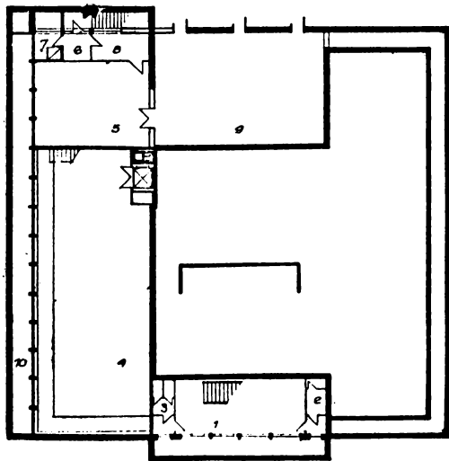
4. ábra. Alagsor
