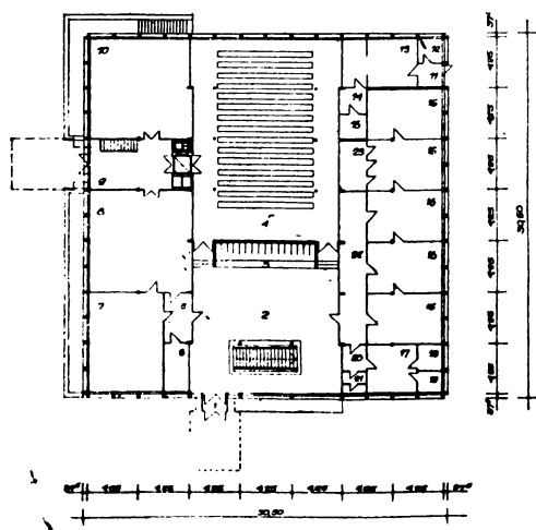
2. ábra. Földszint
