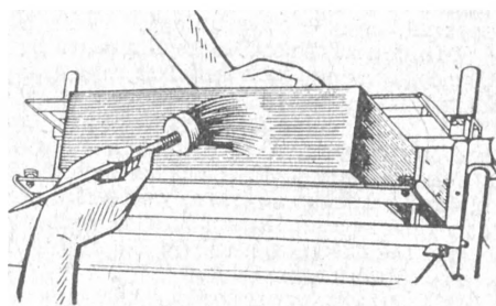
2. sz. ábra. Első kenés
