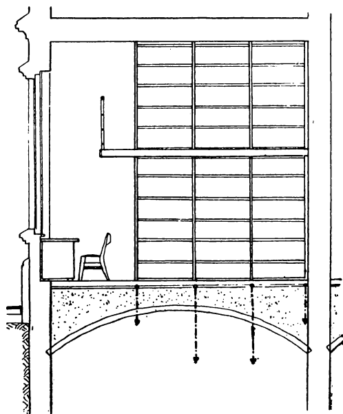
2. sz. ábra. Boltív féloldalas terhelése
