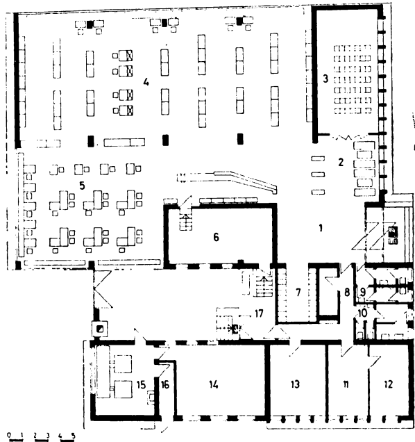
Alaprajz. 1. előtér, 2. lapozgató, 3. előadóterem, 4. könykválasztó, 5. olvasó, 6. könyvraktár, 7. ruhatár, 8. székraktár, 9. mosdó, 10. személyzeti mosdó, 11. hálózati előadói iroda, 12. igazgatói iroda, 13. feldolgozó, 14. tüzelőraktár, 15. káznház, 16. előtér, 17. előtér-csomagoló.
