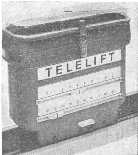
A „Telelift” kocsi a sínen. A szállítódoboz homlokzati részén az elektronikus irányítóberendezés gombrendszere látható. A doboz szállítás közben zárt
