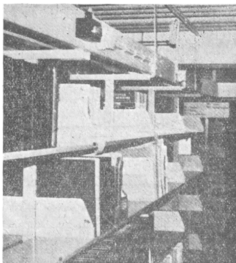
Polcok tetejére szerelt szállítószalag és csatlakozása (jobbról) a fővonalhoz.
