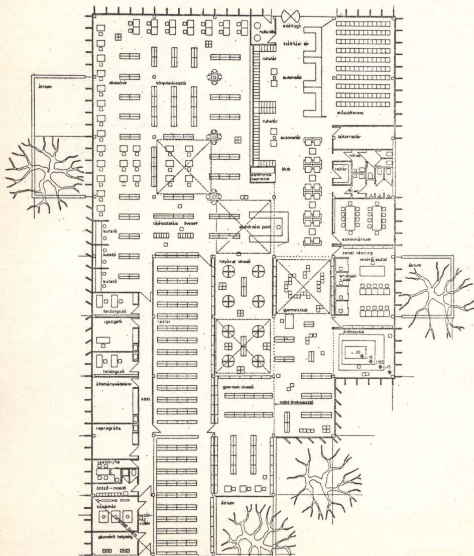
A „Középfokú közművelődési könyvtár” pályázaton III. díjjal jutalmazott munka Gerő Balázs-nak és munkatársainak terve. Különösen építészeti vonatkozásban mutat erényeket. A téglake-rítések mögött rejtőző külső udvarok azonban nincsenek szerves kapcsolatban a belső felada-tokkal, olvasóudvarként ugyanis nem használhatók. Továbbtervezés esetén gondoskodni kell a közösségi terek elhatárolásáról. (Cikkünket ld. a 190. oldalon)
