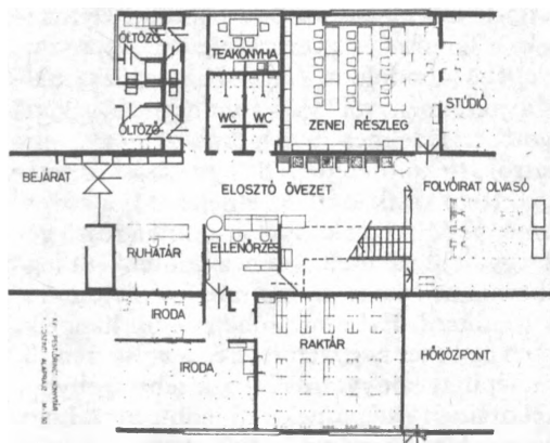
A XVIII. kerületi – pestlőrinci – könyvtár földszinti alaprajza M = 1:50
