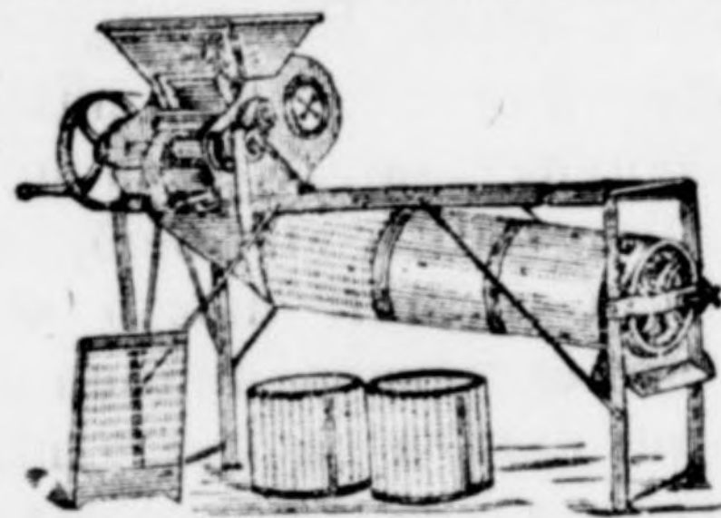
Konkolyozó (Trieur).
