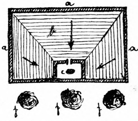
A kiscgazda trágyatelepe felülnézetben
