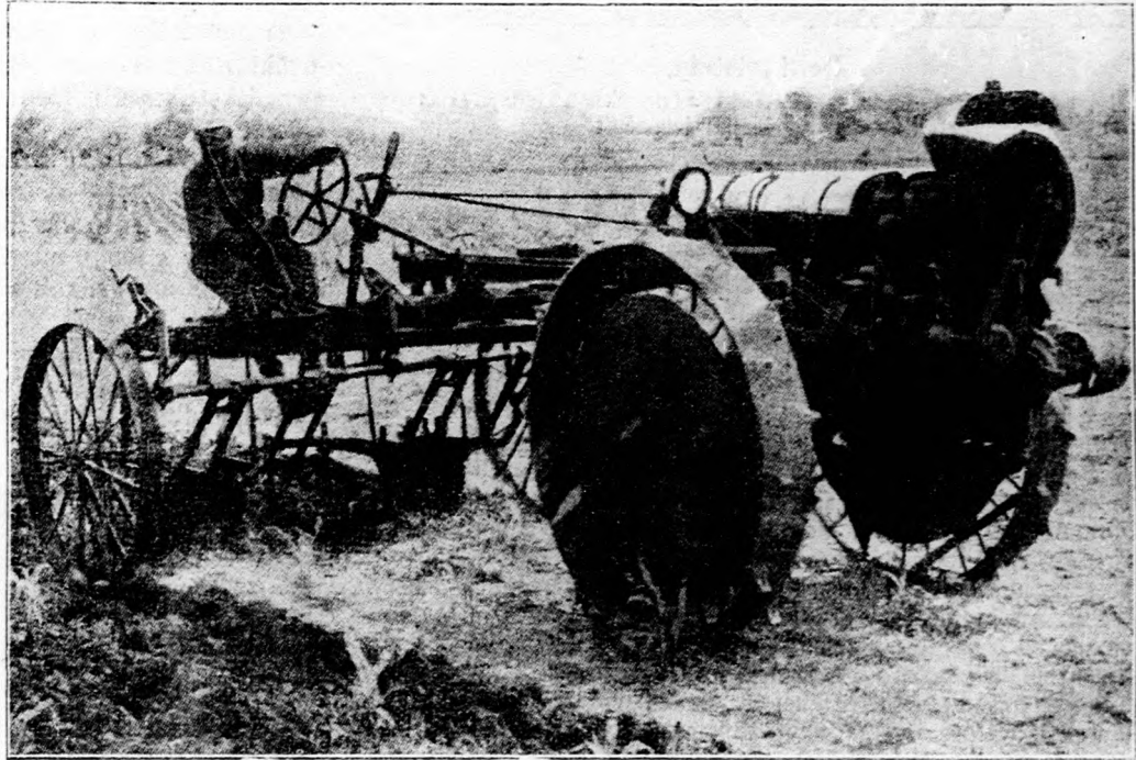
Tengeri kapálás és töltögetés motorral.
