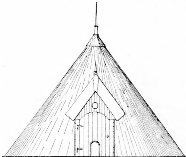
Baromfió. Előlnézet.
