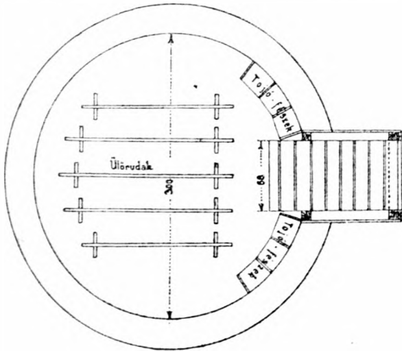
Alaprajz. Az előforduló számok centimétereket jelentenek.
