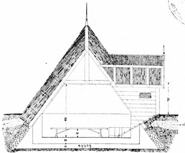
Baromfió. Hosszmetszet.
