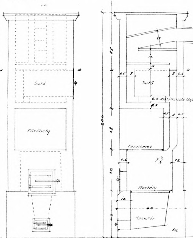
Lengyel kályha.
