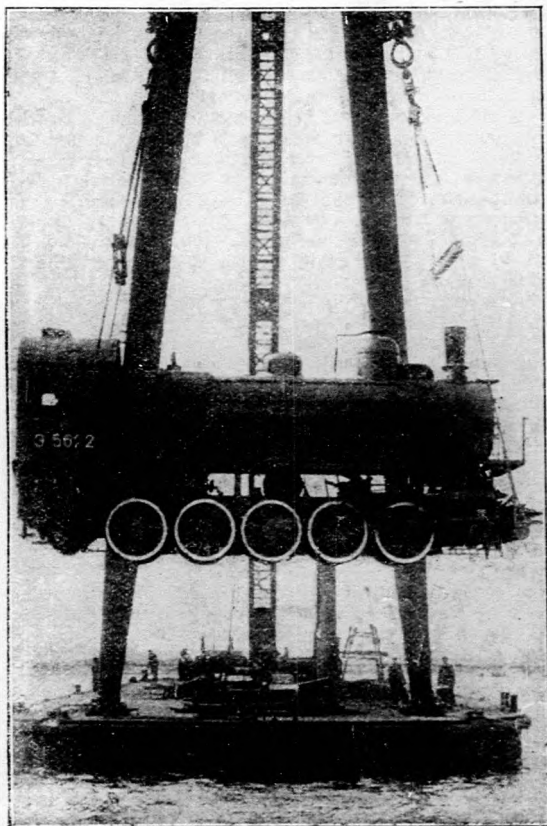
Egy hatalmas mozdony szállítása úszódokk segítségével.
