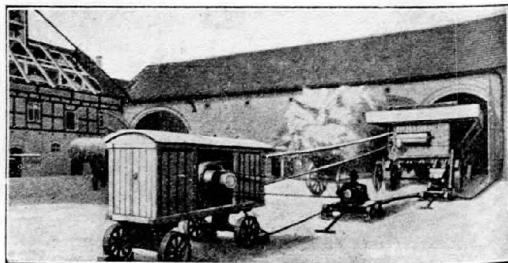
Fúvószerkezet a szemes gabona szállítására.
