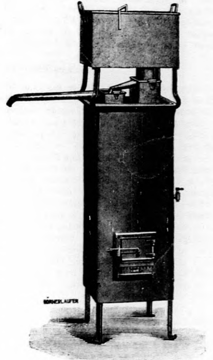
4. „Alfa” tejelőmelegítő és pasztöröző-készülék.
