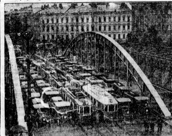
Egy új hid terhelési próbája Bécsben. Két sor villamos, négy sor teherautó; összesen 643 tonna súlyban.
