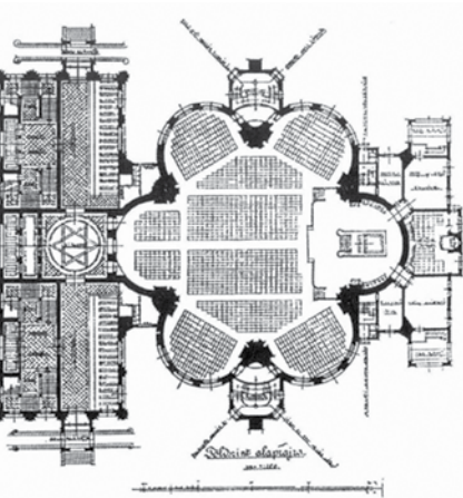
Leitersdorfer (Lajta) Béla zsinagógatervének rajza (Építő Ipar 1899. XXIII. évf. 88. o.)
