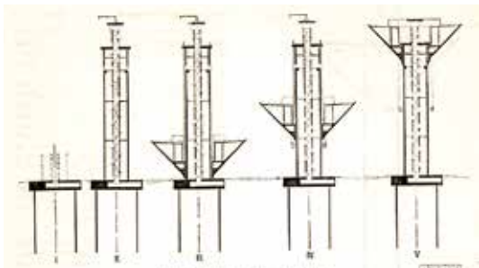
A Lakatos utcai víztorony építési fázisai. Forrás: adt/ Mélyépítéstudományi Szemle, 1990. 1. szám
