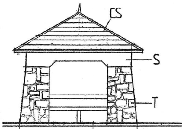
A tervezett buszmegálló keleti homlokzata
