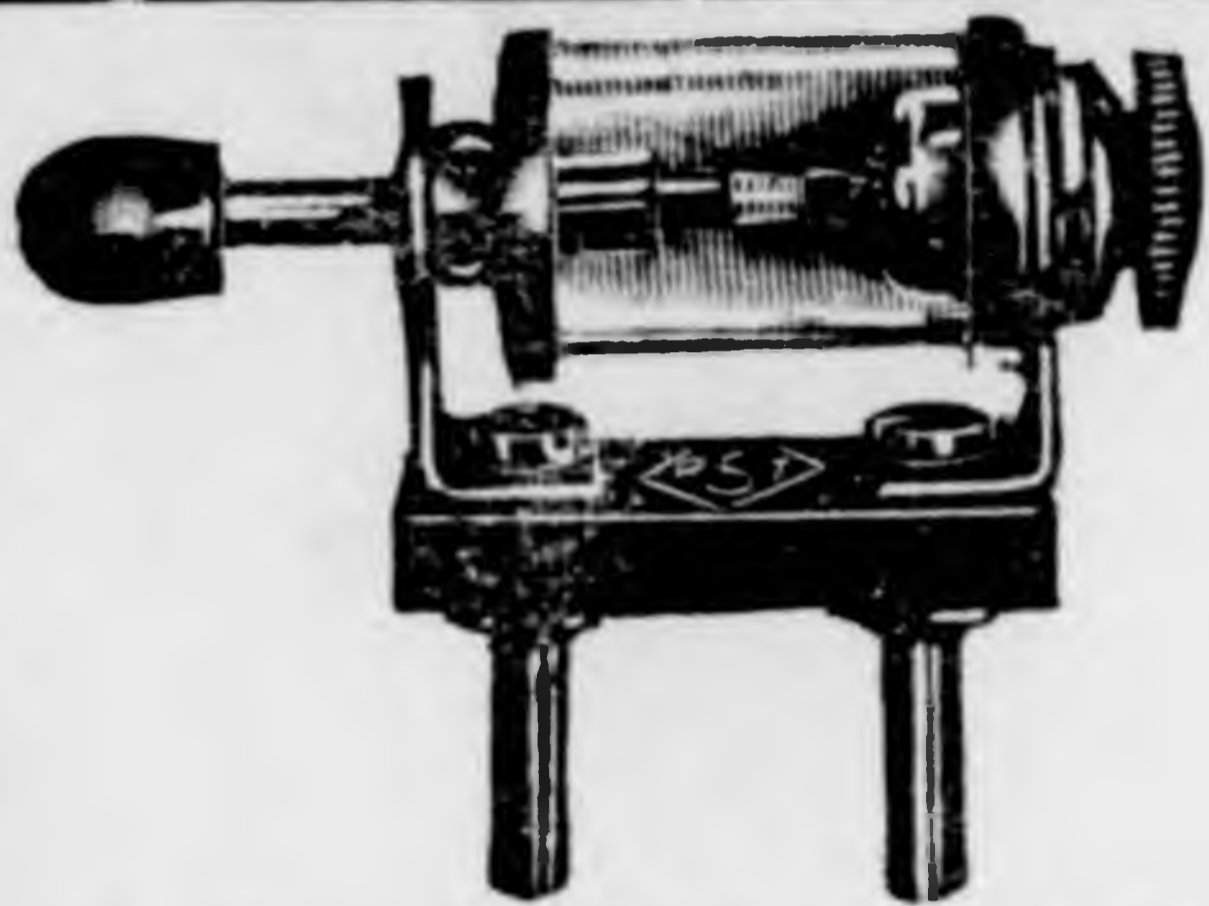
S. R. T. „ROYAL” defektor Legprecízebb kivitel, nagyon érzékeny, hangerős kristállyal, mely azonnal kicserélhető, legolcsóbb ár
