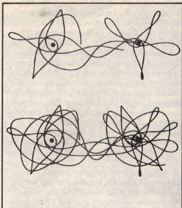
Két csillag körül keringő bolygó pályája: példa a kaotikus viselkedésre. Ha bevezetjük a súrlódást, sokkal kellemesebb képet kapunk (ez az ún. Lorenz-attraktor).
