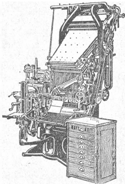
Linotype négymagazinos soröntő szedőgép
