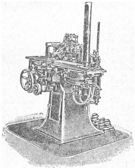
A monotype szedőgép öntőgépe
