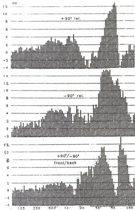
10. ábra: Az elől-hátul érzékelés kimutatása +90^\circ és -90^\circ relatív szinképeinek kivonásával. Részletek a szövegben
