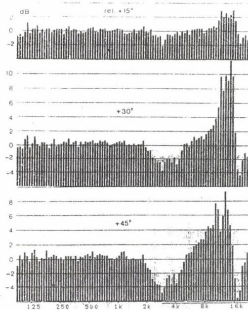
6. ábra: Relatív (a 0^\circ irányú színeképből kivont) színeképek pozitív ferdeszögű irányokból. Megjegyzendő, hogy a negatív dB-értékek intenzitás-gyarázkodást, a pozitívok intenzitás-gyengülést jelentenek az illető irányban
