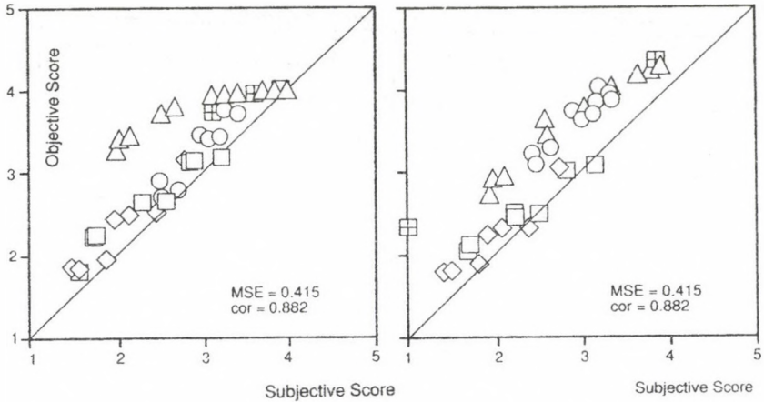
A szubjektív és az objektív értékelés kapcsolata a PSQM módszerek alkalmazásával
