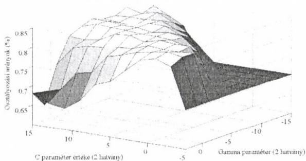
3. ábra Az SVM optimalizálása 12 MFC esetén
