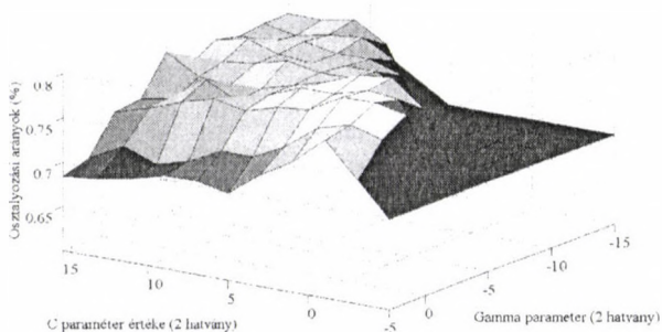
4. ábra Az SVM optimalizálása 12 MFC + \Delta + \Delta\Delta esetén
