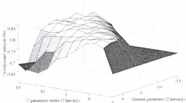
5. ábra Az SVM optimalizálása 24 MFC esetén
