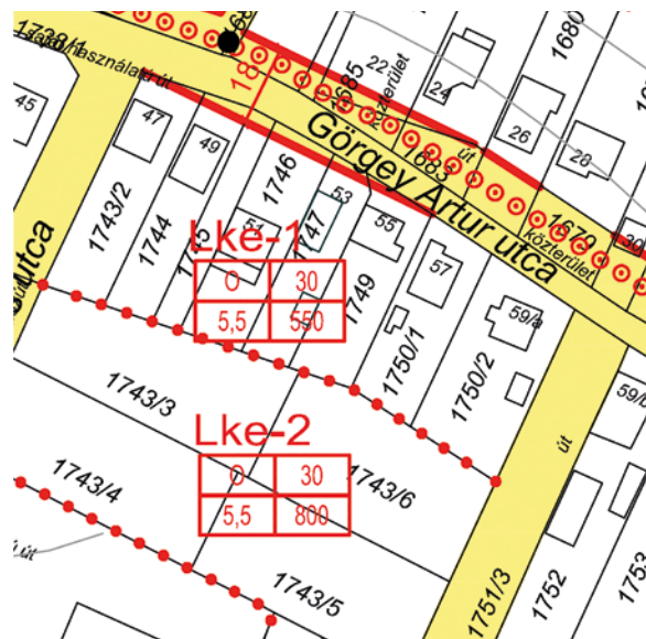
Jellemző részlet a szabályozási tervből
