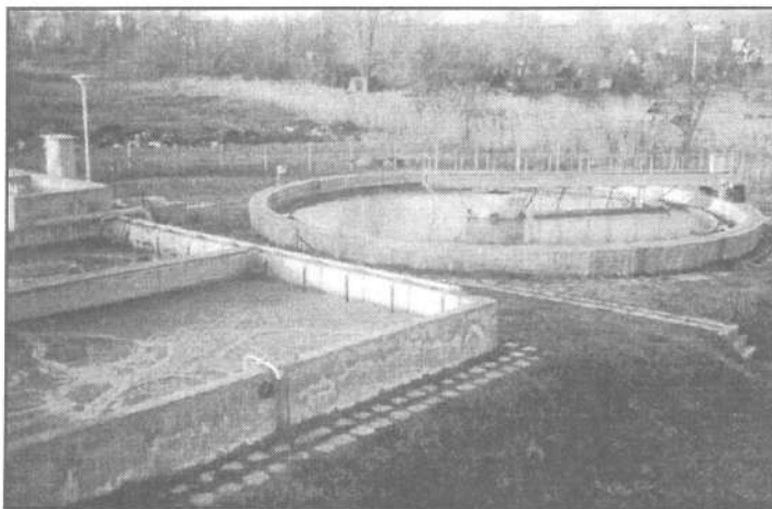
Az eleveniszapos medence és a kör alakú utóülepítő
