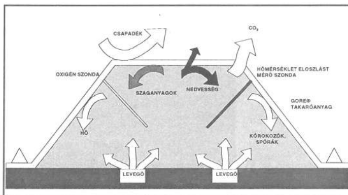
A komposztáló prizma működési elve
