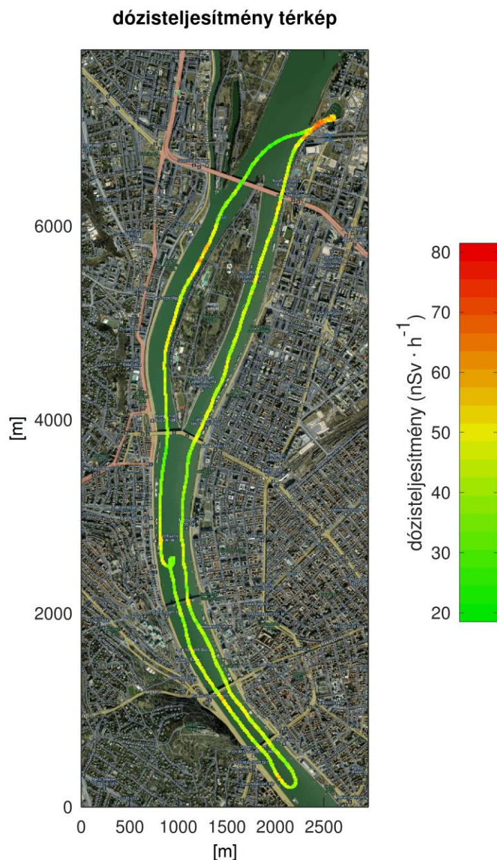
3. ábra. Dózisteljesítmény térkép a folyami sugárfelderítésről
