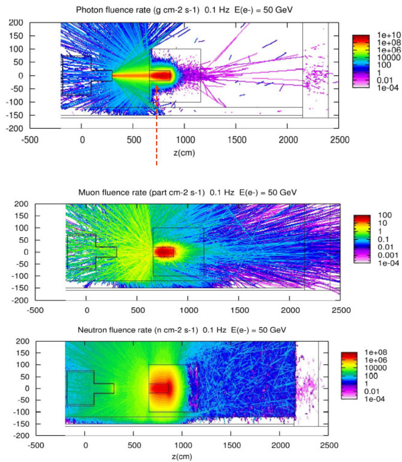
7. ábra: A nyaláb csapda tovább fejlesztett változata, grafit rúddal a közepén. A jobb oldalon van a részecske fluensteljesítmény színskódja ( \text{részecske.cm}^{-2}\text{s}^{-1} ), az y és z tengelyen a távolság saválló acélban (cm).
