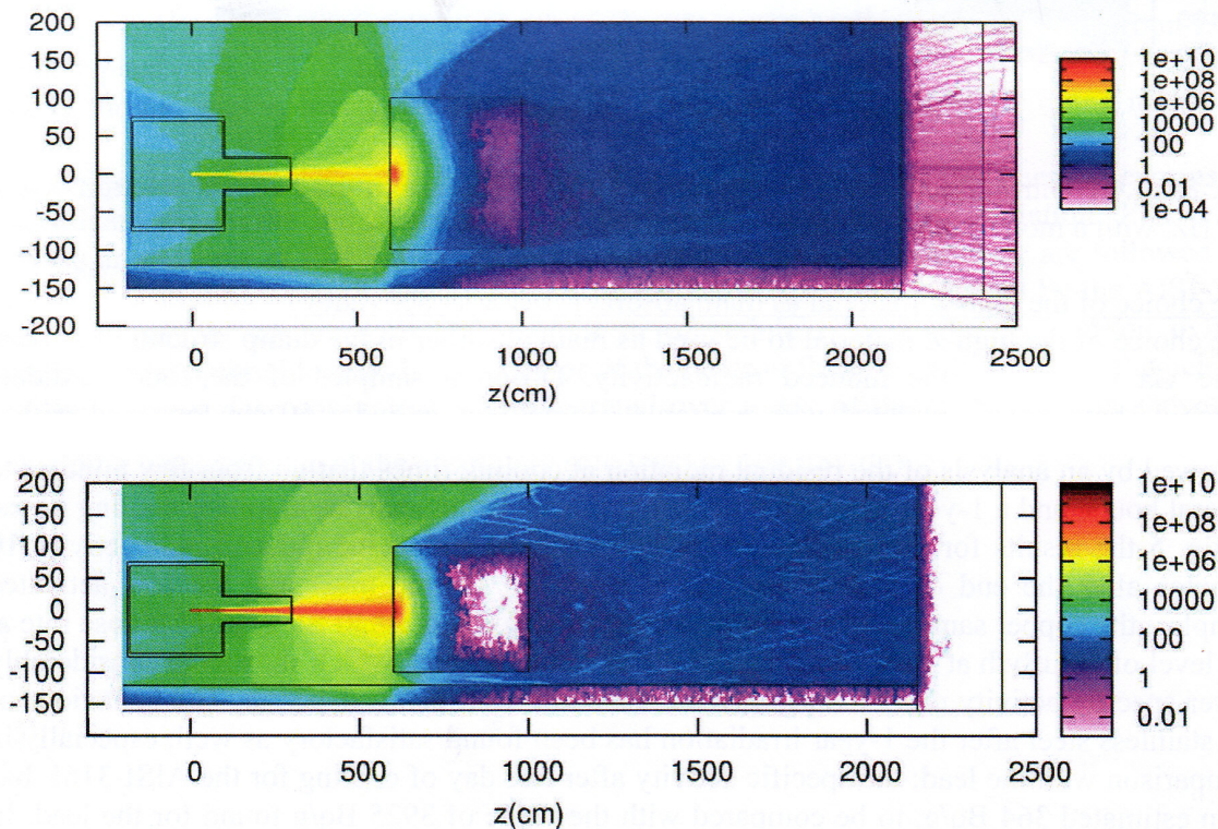
6. ábra: A környezeti dózisegyenérték-teljesítmény 50, illetve 5 GeV-os elektron nyaláb esetén. A jobb oldalon van a környezeti dózisegyenérték-teljesítmény színskódja ( \mu\text{Sv/h} ), az y és z tengelyen a távolság saválló acélban (cm).
