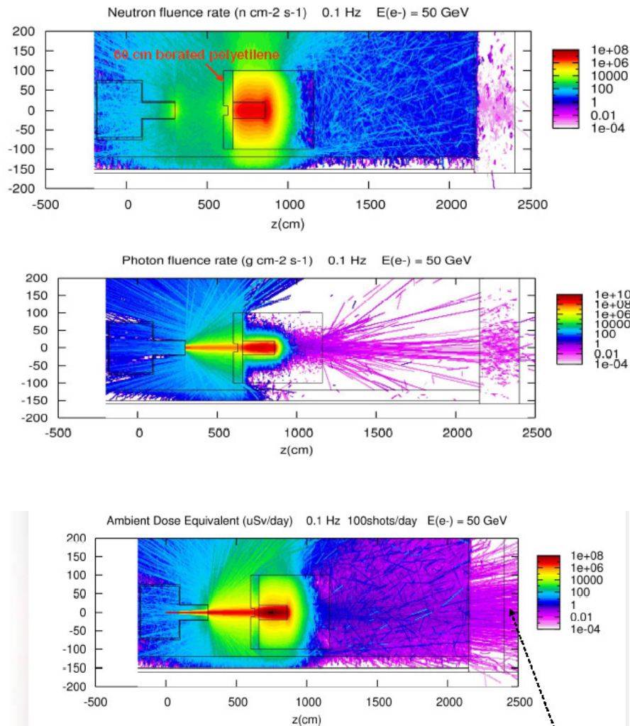
8. ábra: A nyaláb csapda bórozott polietilénnel kiegészítve. Az első két ábrán a színekód a részecske fluensteljesítmény (részecske.cm -2 s -1 ), az y és z tengelyen a távolság saválló acélban (cm). A harmadik ábra jobb oldalán a színekód a környezeti dózisegyenérték-teljesítmény (μSv/nap).
