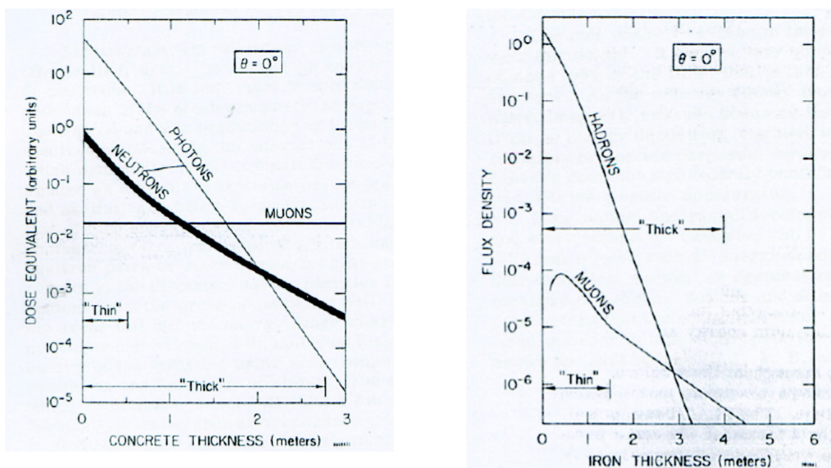
3. ábra: A müon sugárzás hatékony árnyékolása vasból készült falakkal (jobb oldali ábra), a beton gyakorlatilag nem gyengíti a sugárzást (bal oldali ábra) [2]
