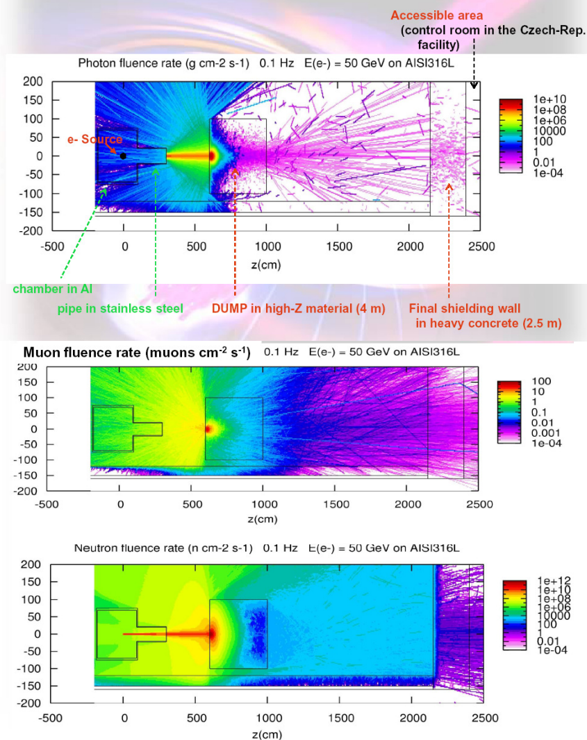
5. ábra: 50 GeV-os elektron nyaláb által keltett másodlagos sugárzások okozta részecske fluensteljesítmény eloszlás. Az y és z tengelyen a távolság a saválló acélban (cm), jobb oldalon a fluensteljesítmény színskódja ( \text{részecske} \cdot \text{cm}^{-2} \text{s}^{-1} ).
